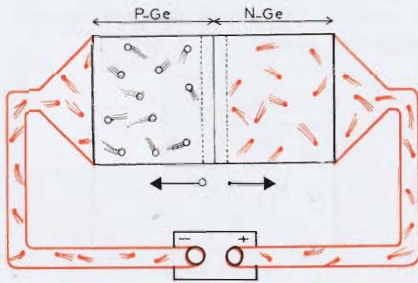
Fig. 16. Diode geschakeld in keerrichting.
