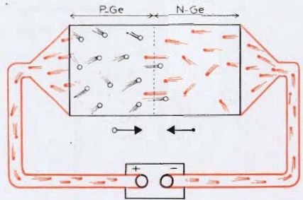
Fig. 17. Diode geschakeld in doorlaatrichting.
