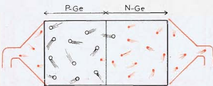
Fig. 14. Grensverkeer van de vrije elektronen en gaten.
